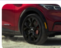
Leichtmetallrad 19" 5-Speichen-Y-Design, Ebony Black 7 x 19", ET 47,5, für Reifengröße 225/55 R19
