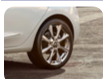
Jante en alliage 18" Modèle 8 branches, poli 7 x 18", déport 47.5, pour pneus 205/40 R18
