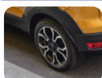
Jantă din aliaj 17" design cu 5 x 2 spițe, Negru absolut prelucrat 7 x 17", offset 37,5, pentru anvelope 205/50 R17
